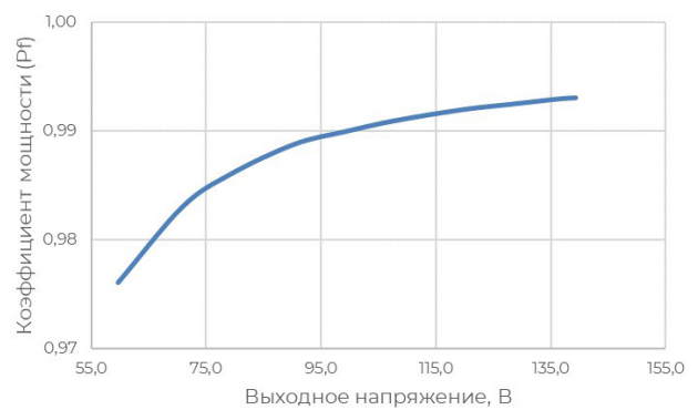
Рис. 2 - Зависимость коэффициента мощности от выходного напряжения
