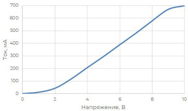
Рис. 5 - Зависимость выходного тока от напряжения диммирования
