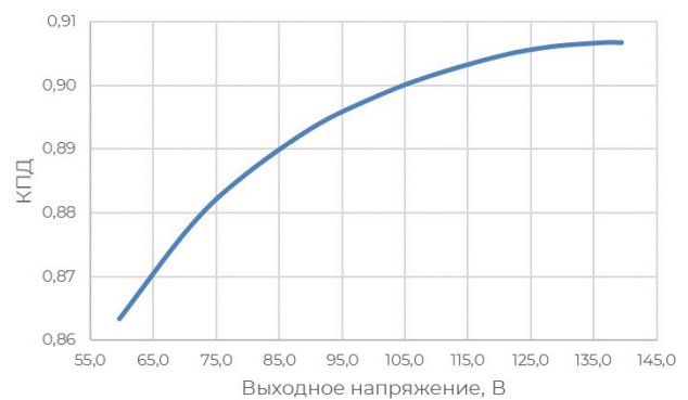
Рис. 4 - Зависимость КПД от выходного напряжения
